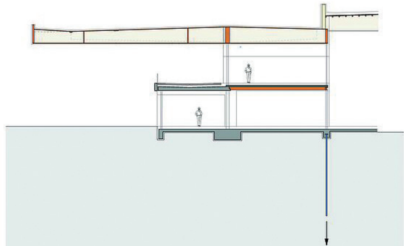
Querschnitt des Vordachs: Die knapp 28 m langen Dachelemente mit 18,60 m großer Auskragung werden in der 9,30 m zurückliegenden Gebäudeachse zurückgespannt. (Quelle: merz kley partner)
